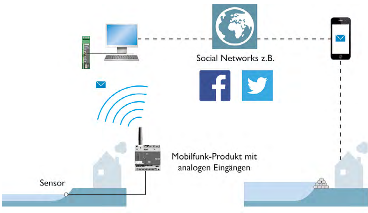
Abbildung 7: Wasserstandfrühwarnsystem zum Hochwasserschutz
