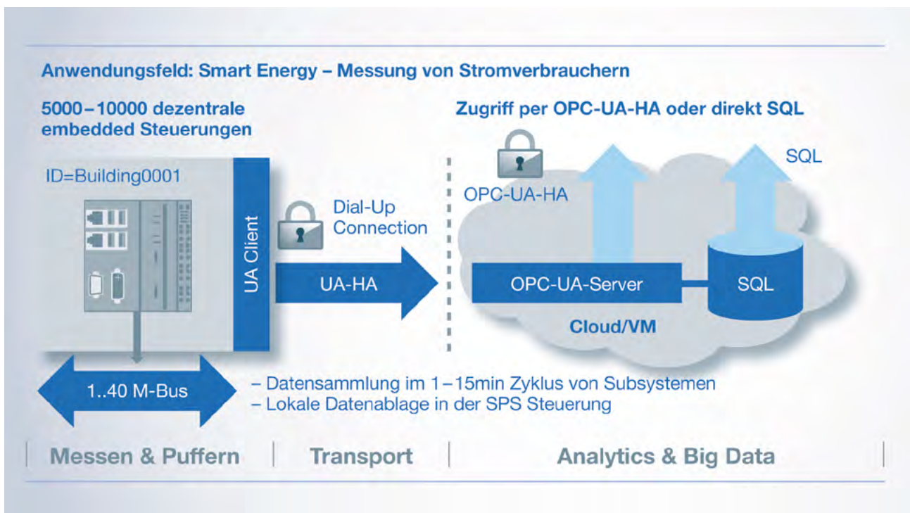
Abbildung 3: Smart Energy – Messung von Stromverbrauchern
