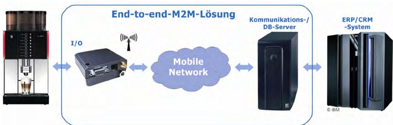
Abbildung 6: Telemetrie gewerblicher Kaffeemaschinen
