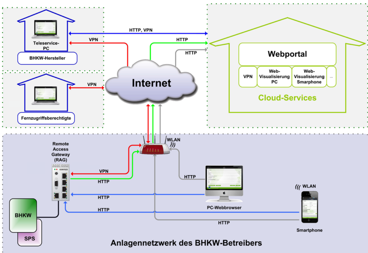
Abbildung 1: Fernzugriff und Fernsteuerung für Blockheizkraftwerke
