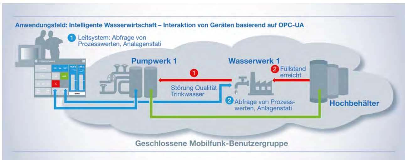
Abbildung 2: Intelligente Wasserwirtschaft – Interaktion von Geräten
